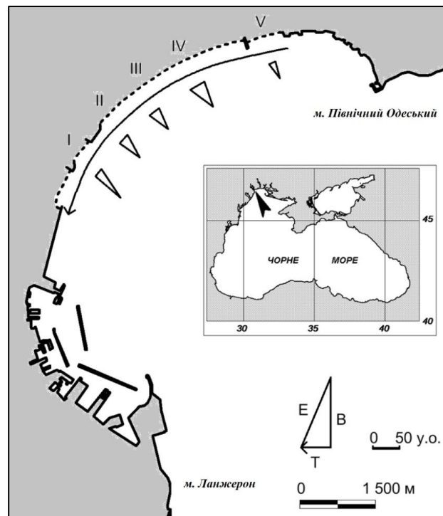
Рис. 2. Схема розподілу хвиленергетичних характеристик ( E , B , T_{рез} ) вздовж берегу Одеської затоки (положення вказано стрілкою на врізці)
